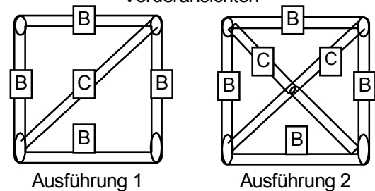
Vorderansichten
